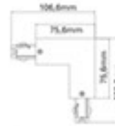
MA 05-Right L Feed Part MA 05-Sağ L Bağlantı MA 06-Left L Feed Part MA 06-Sol L Bağlantı
