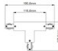
MA 09-Right T Corner Part MA 09-Sağ T Köşe Bağlantı MA 10-Left T Corner Part MA 10-Sol T Köşe Bağlantı
