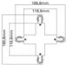
MA 07-X Feed Corner Part MA 07-X Bağlantı Elemanı
